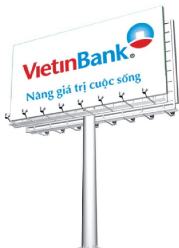
Kích thước mặt biển: * 20m(dài) x 10m(rộng) x 2mặt * 15m(dài) x 8m(rộng) x 2mặt Chiều cao từ chân cột tới đỉnh biển: 25m
